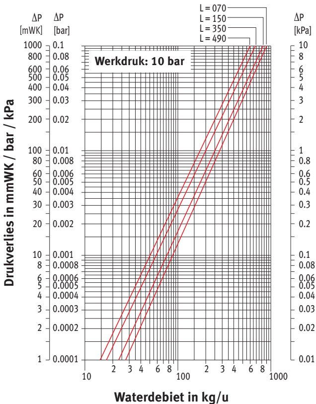
DRUKVERLIES TYPE 19
