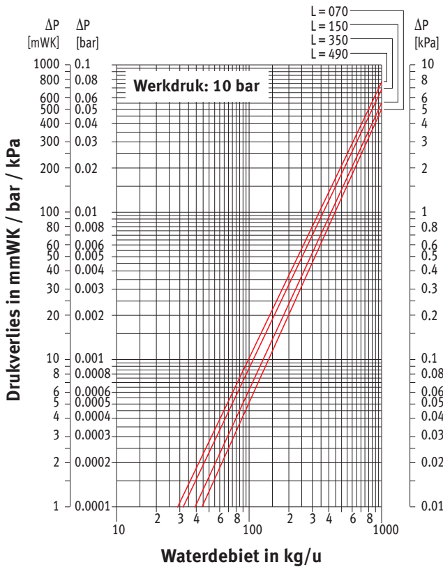
DRUKVERLIES TYPE 20
